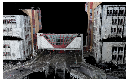
автоматически очищенное облако точек
